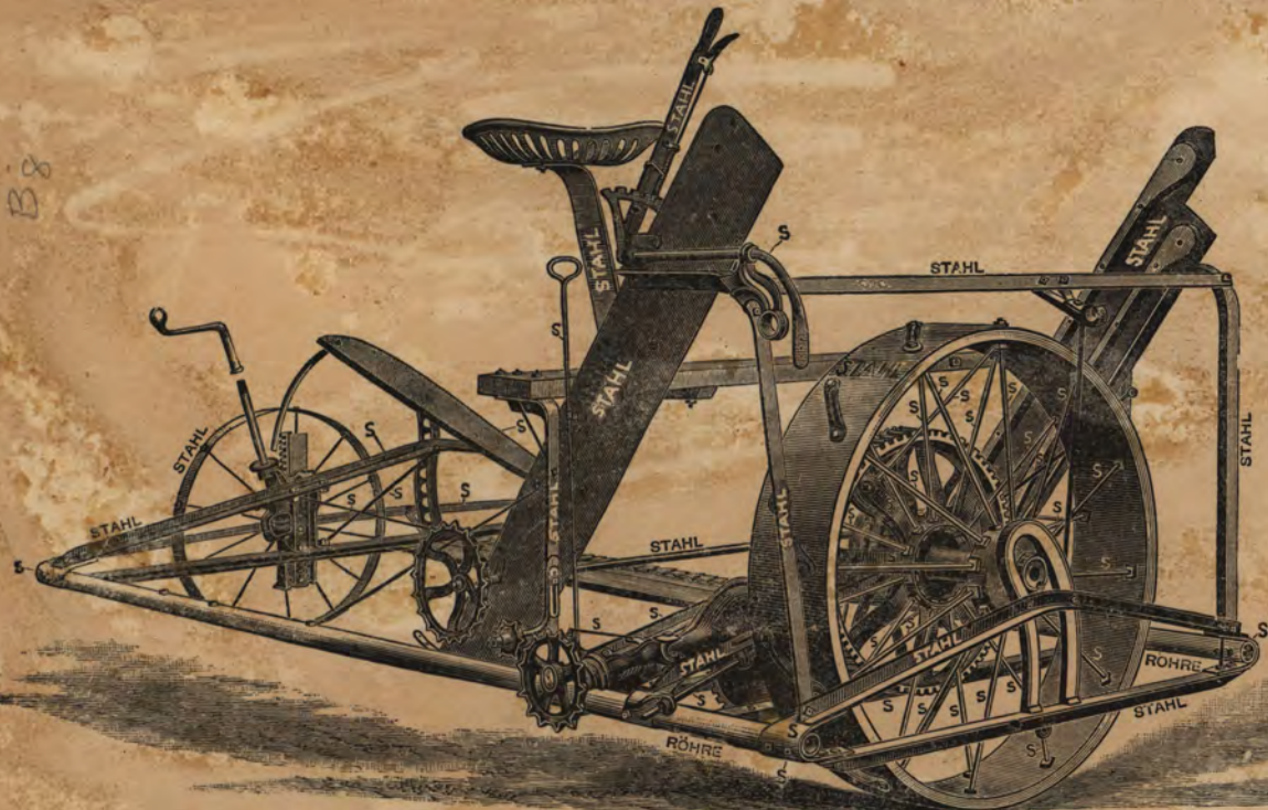
Der Harvester am Deering ganz stählernen Binder — die aus Stahl gemachten Theile zeigend. Die mit "S" bezeichneten Theile sind von Stahl.
